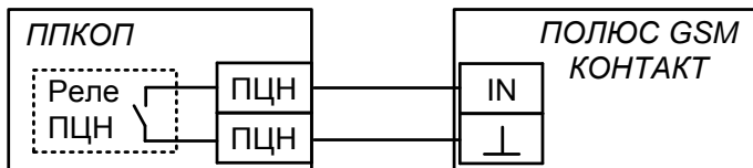
Рис.7 Схема подключения к реле ПЦН ППКОП
