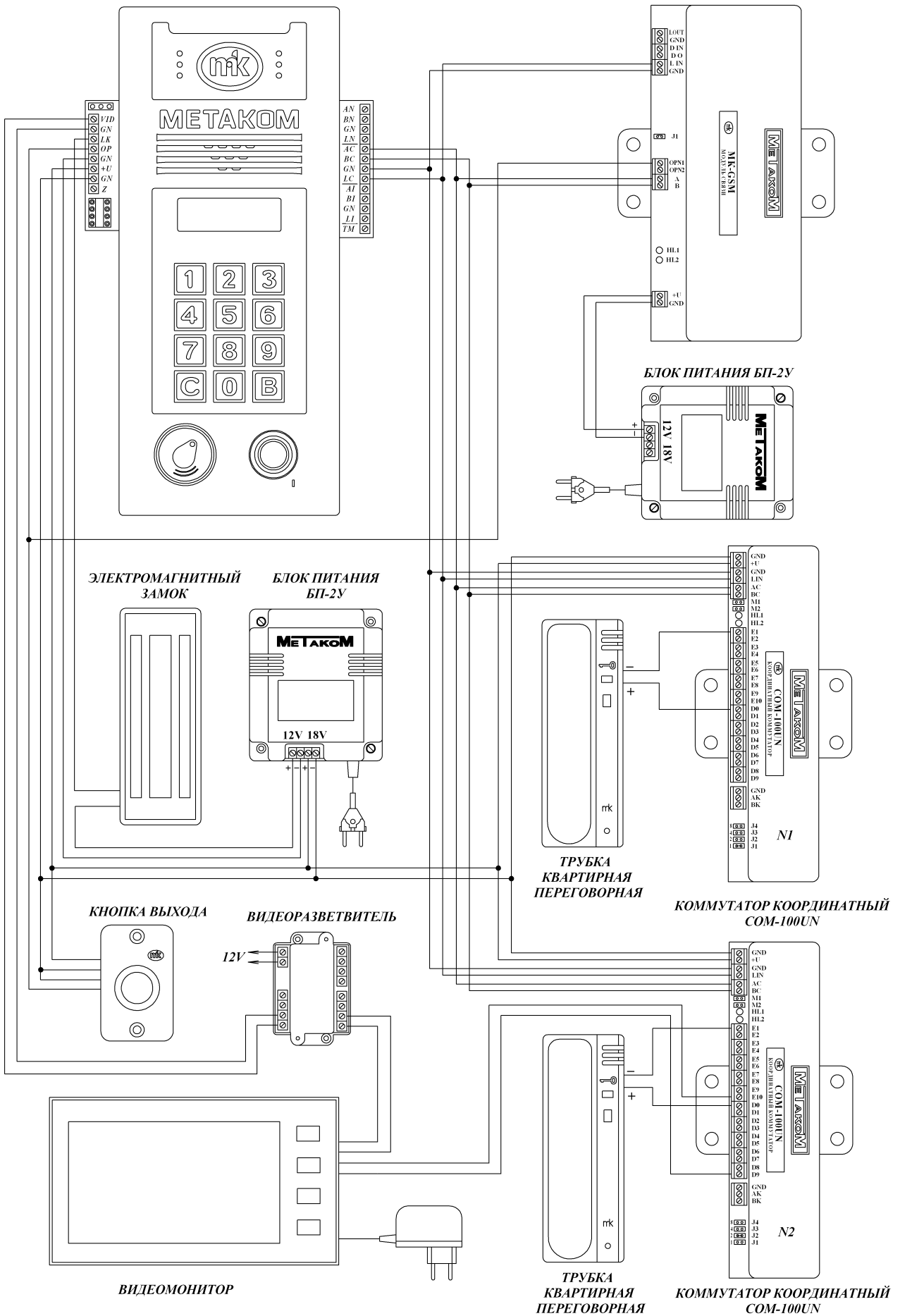
Рис. 2 Пример монтажа блока вызова МК2018-TMRFV
