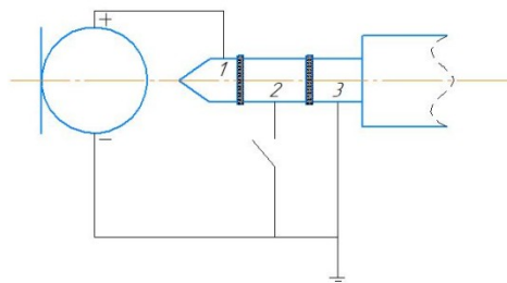
Рис.2. Внутренняя схема подключения
