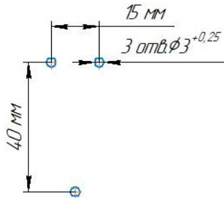
Рис.1 Схема крепления на корпусе изделия
