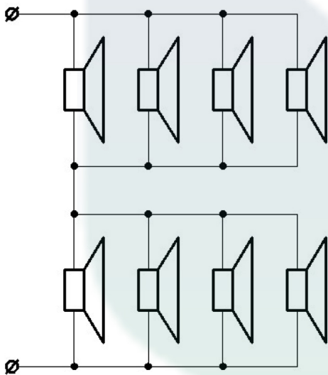
Подключение восьми акустических оповещателей С-3/С-5 8 Ом, R_{\text{вых}}=1,87\text{Вт}/\text{оповещатель}
