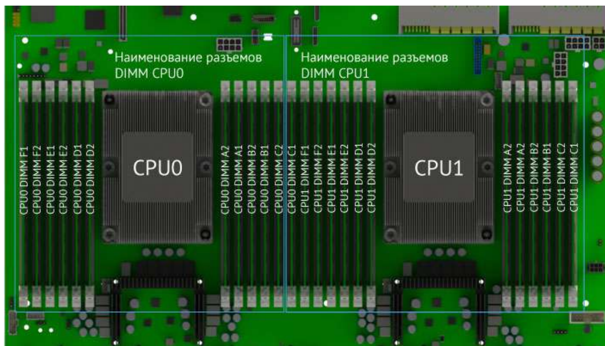
Рис. 33. Расположение разъемов.
