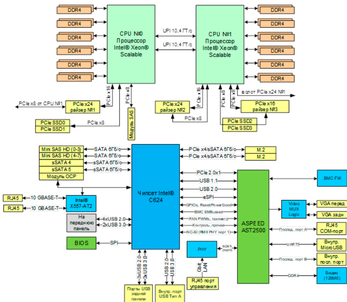
Рис. 1. Структурная схема материнской платы НИКА.469555.001
