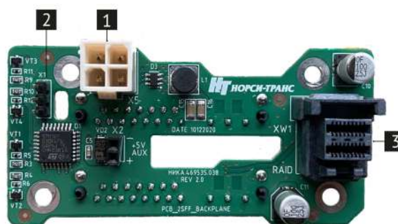
Рис. 15. Плата расширения 2SFF (НИКА.469535.038)
