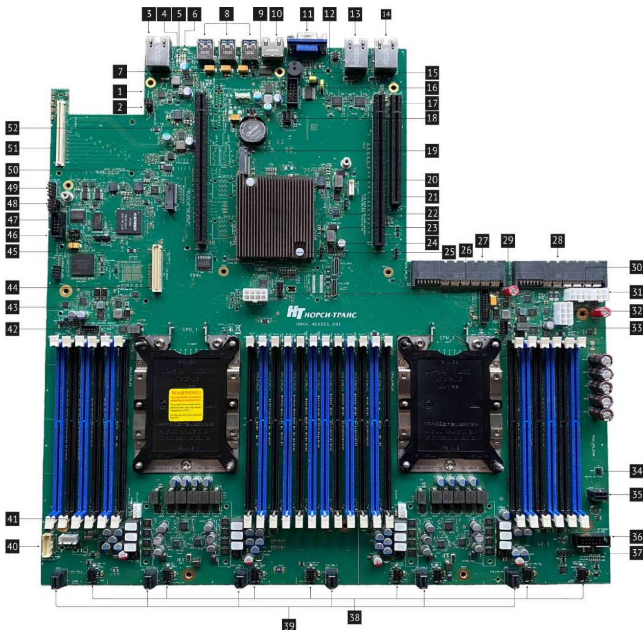
Рис. 13. Соединители и переключатели материнской платы
