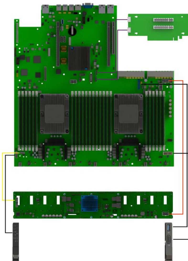
Рис. 30. Схема прокладки системных кабелей и кабелей OcuLink только в случае подключения Райзера 3x16-8-8 (НИКА.469535.047)
