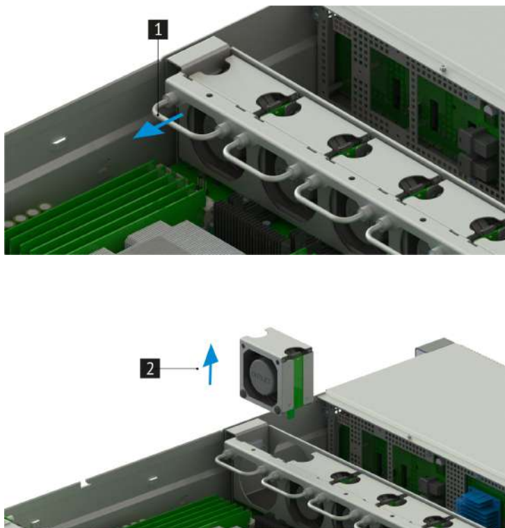
Рис. 31. Извлечение вентилятора.
