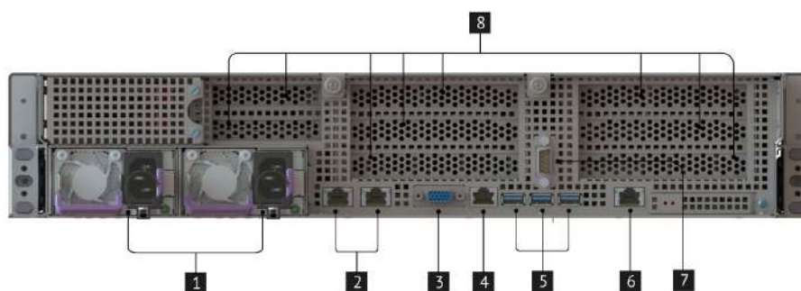
Рис. 4. Вид сервера сзади
