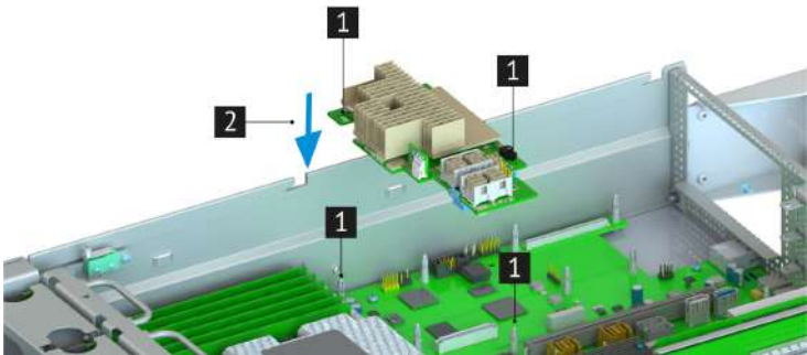
Рис. 46. Установка наплатного RAID-контроллера
