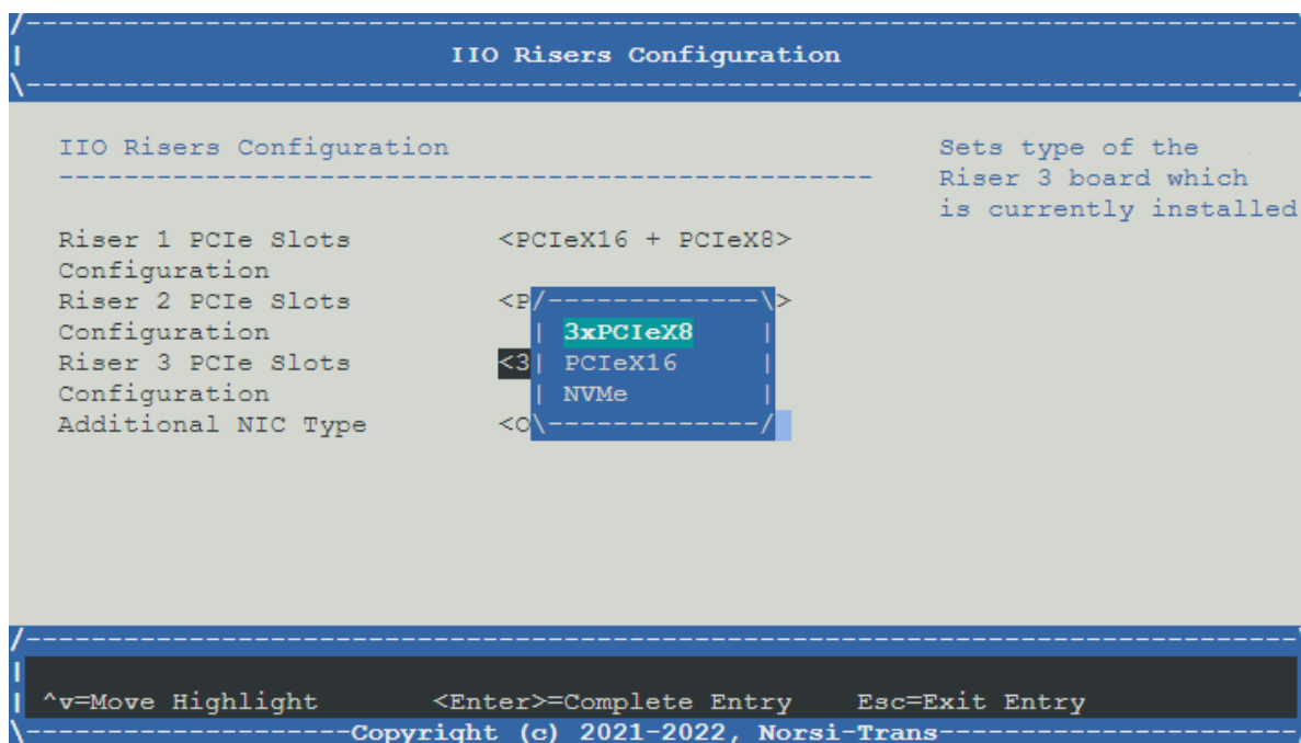
Рис. 68. Выбор типа PCIe-райзеров
