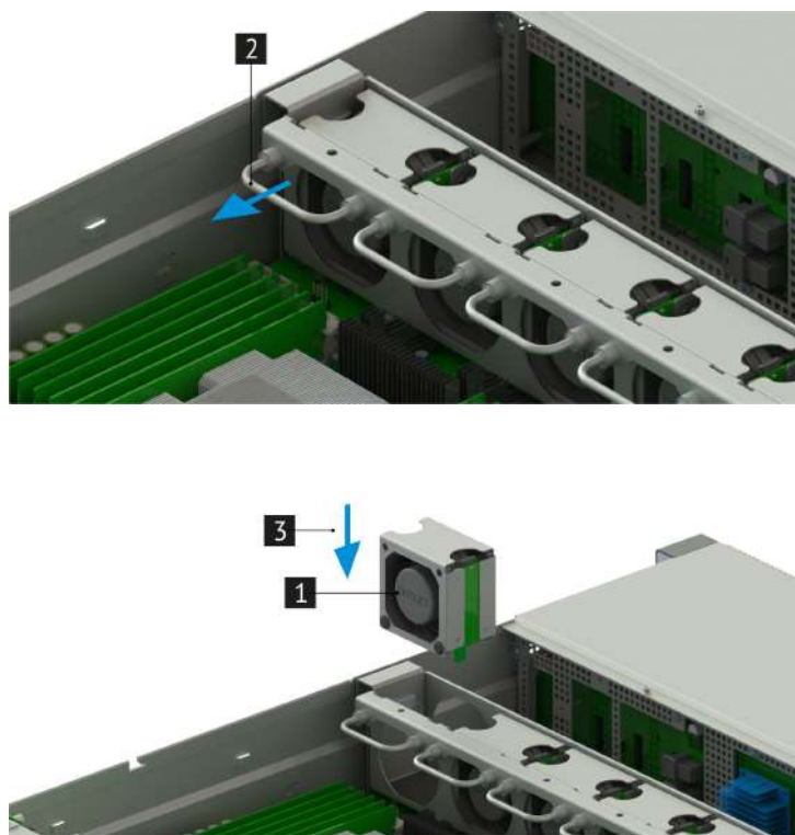
Рис. 32. Подключение вентилятора.
