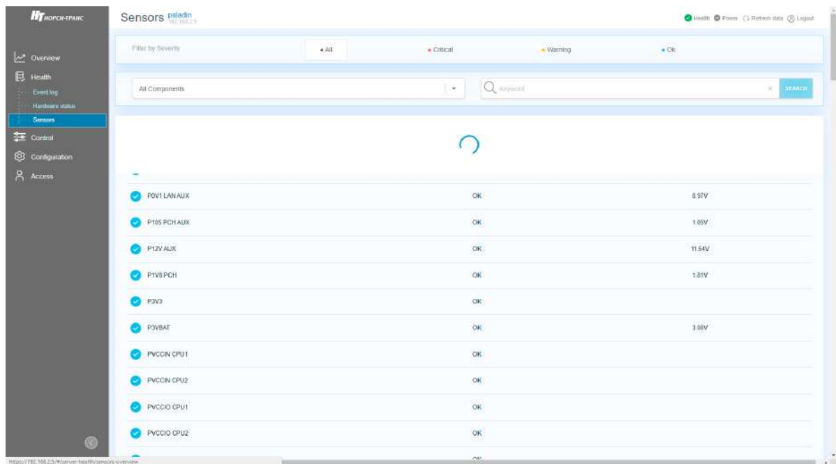
Рис. 71. Окно «Sensors»
