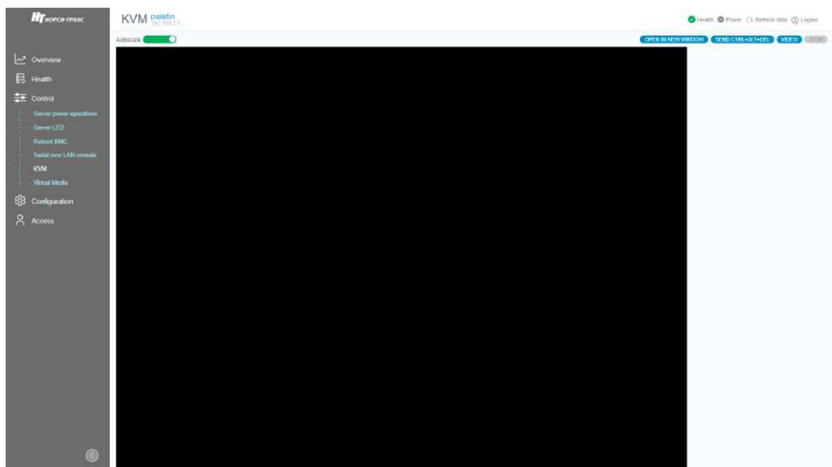
Рис. 76. Окно «KVM»
