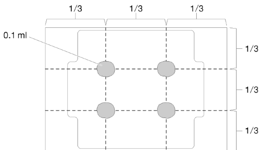
Рис. 39. Нанесение термопасты
