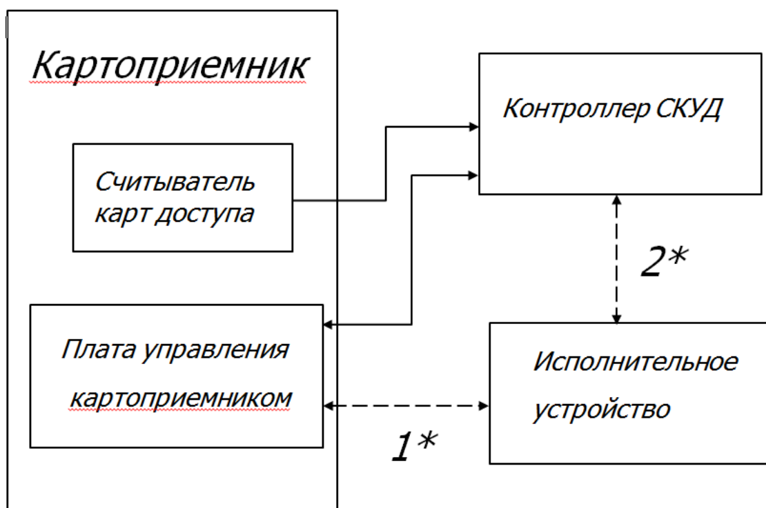
Рисунок 12 – Структурная схема №3
