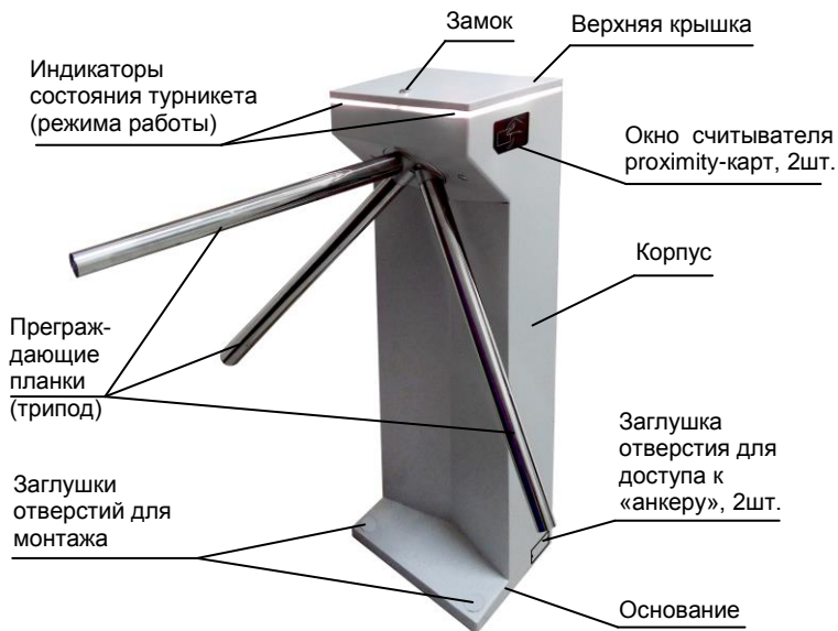
Рис.1 Общий вид турникета
