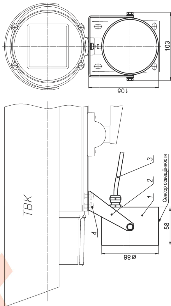
Рис.1 Габаритные размеры и состав изделия
