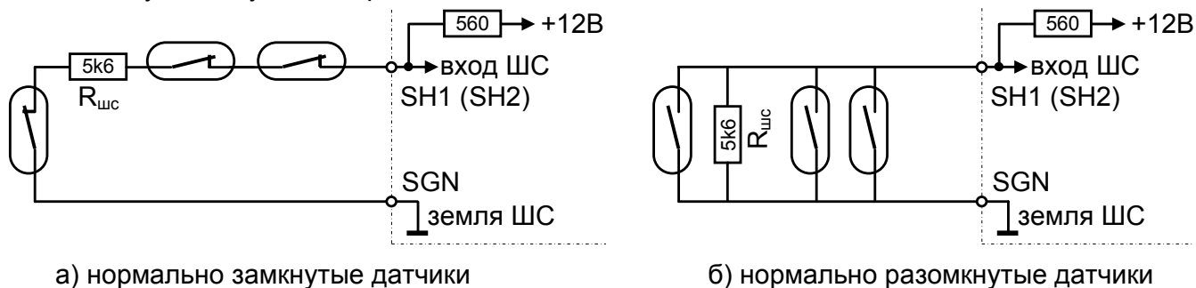
Рис. 2. Примеры монтажа шлейфов сигнализации
