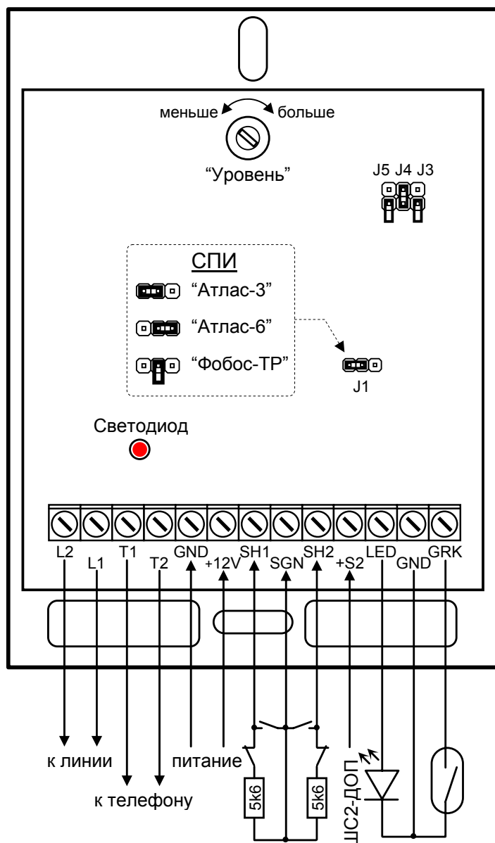
Рис. 4. Монтажная схема устройства исполнения “Риф Бастион-1-Ф”
