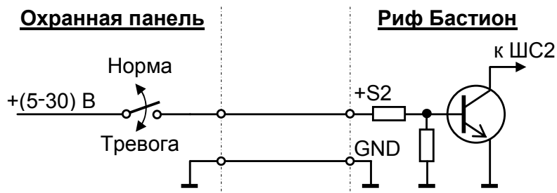
Рис. 3. Пример монтажа шлейфа ШС2-ДОП
