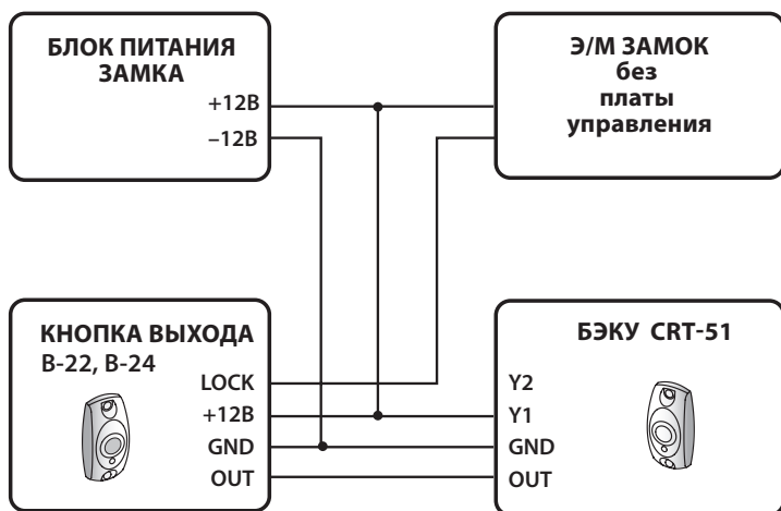
Рис.3 Схема подключения CRT-51 к замку без платы управления и кнопке выхода B-22(B-24)
